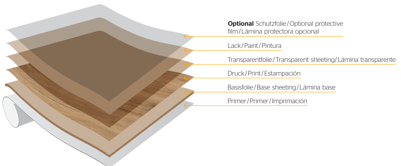
Mehrschicht- (Druckdekor-)Folie / Multilayer (print design) film / Lámina multicapa (estampado decorativo)
